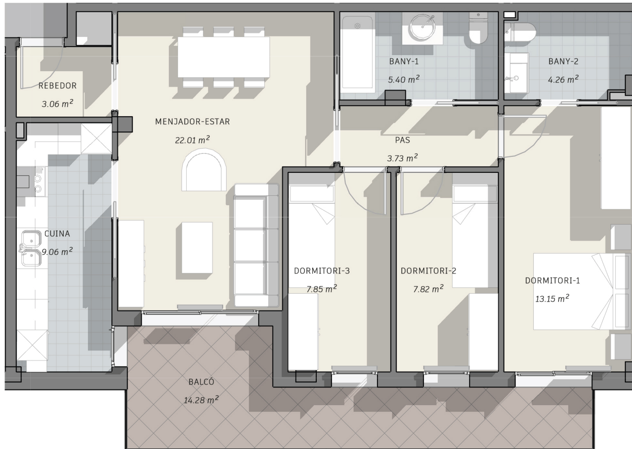
Planta habitatge 2r 5a E= 1:75
